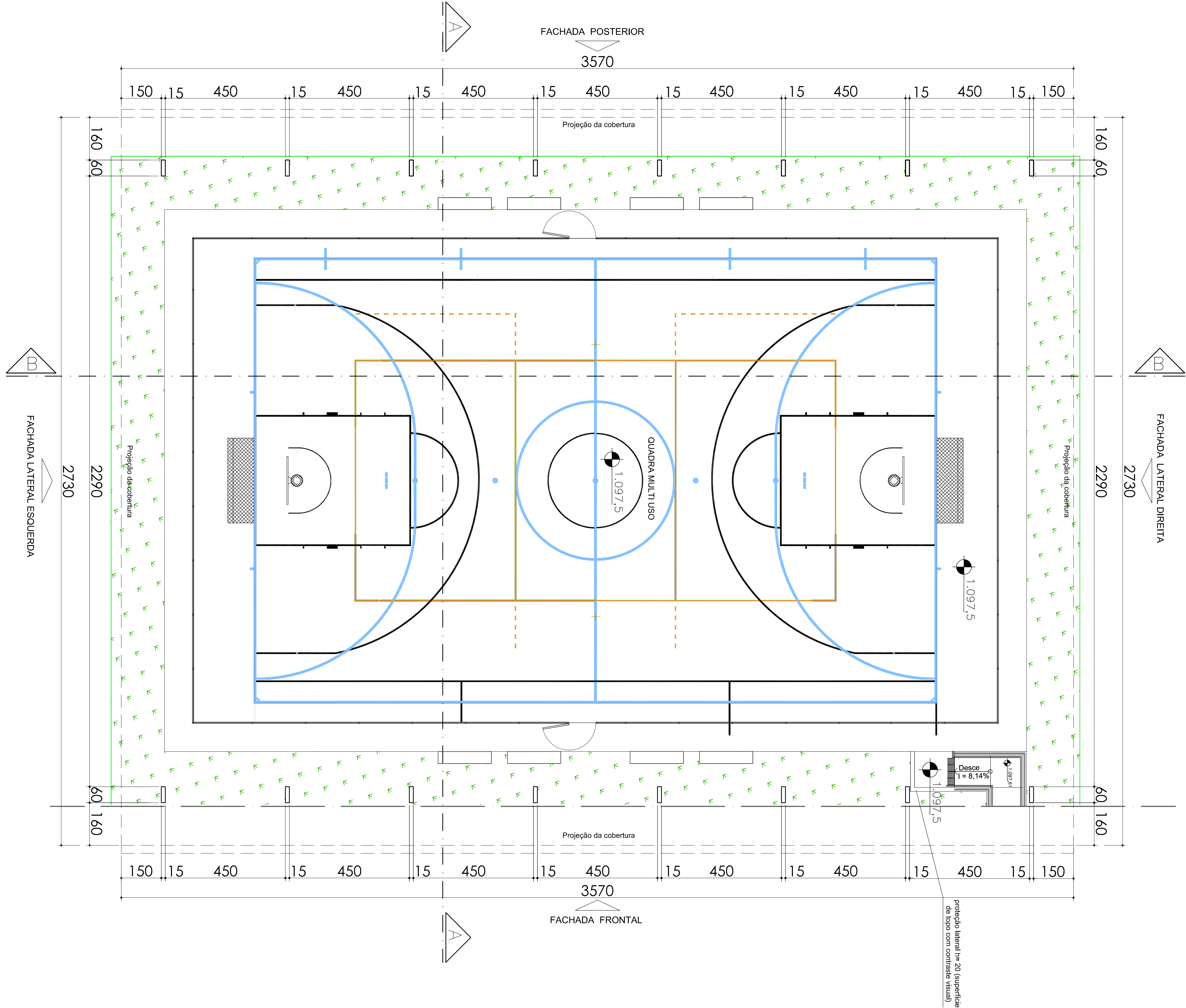
PLANTA - QUADRA POLIESPORTIVA ESC: 1 : 75
