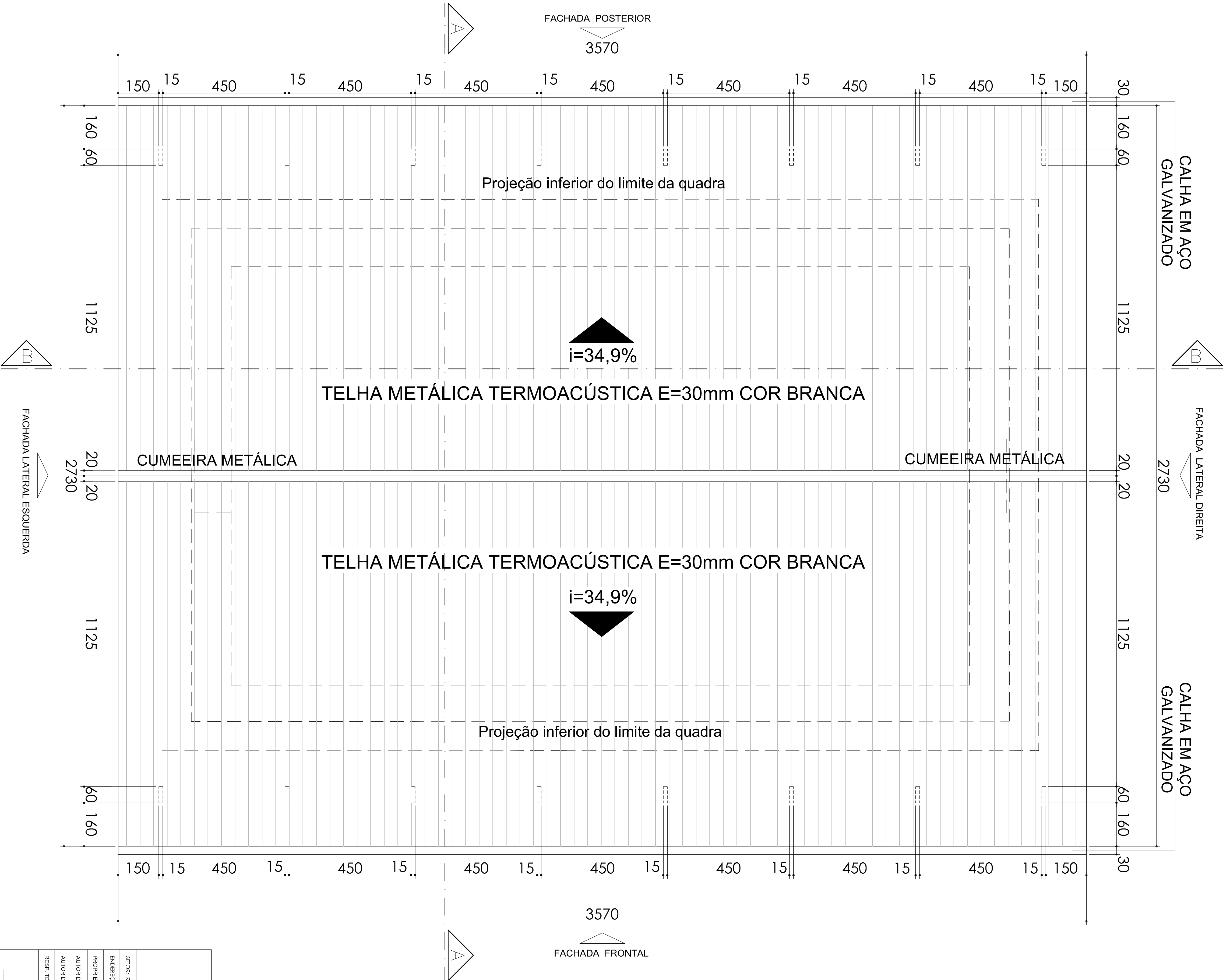
PLANTA DE COBERTURA ESC: 1 : 75
