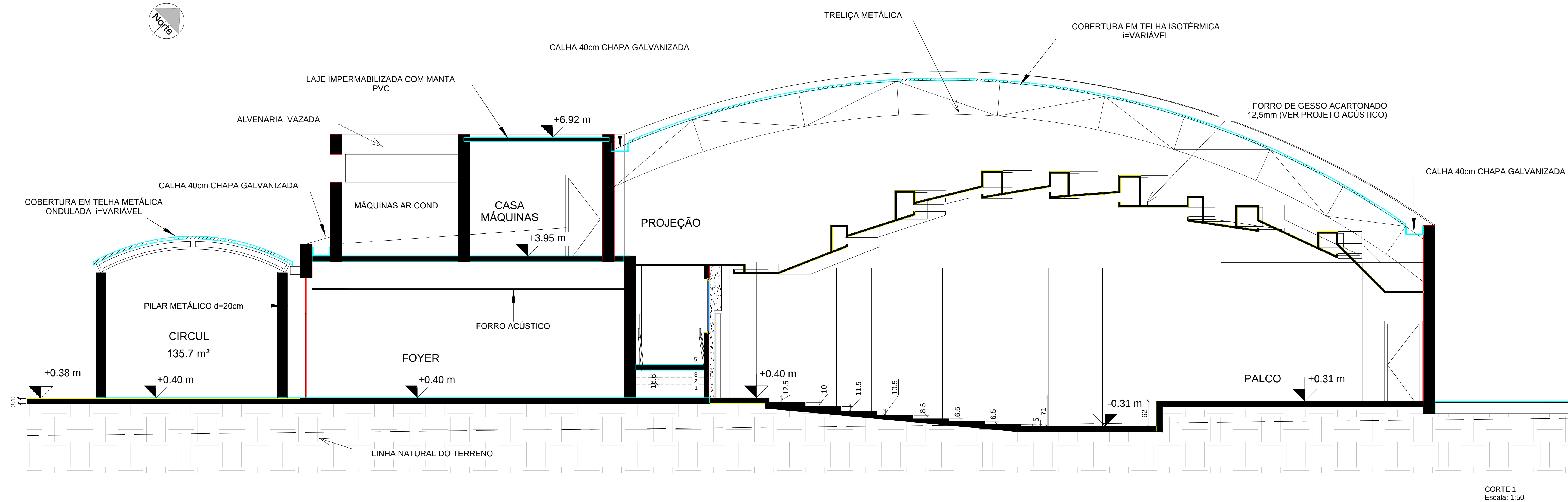
CORTE 1 Escala: 1:50
