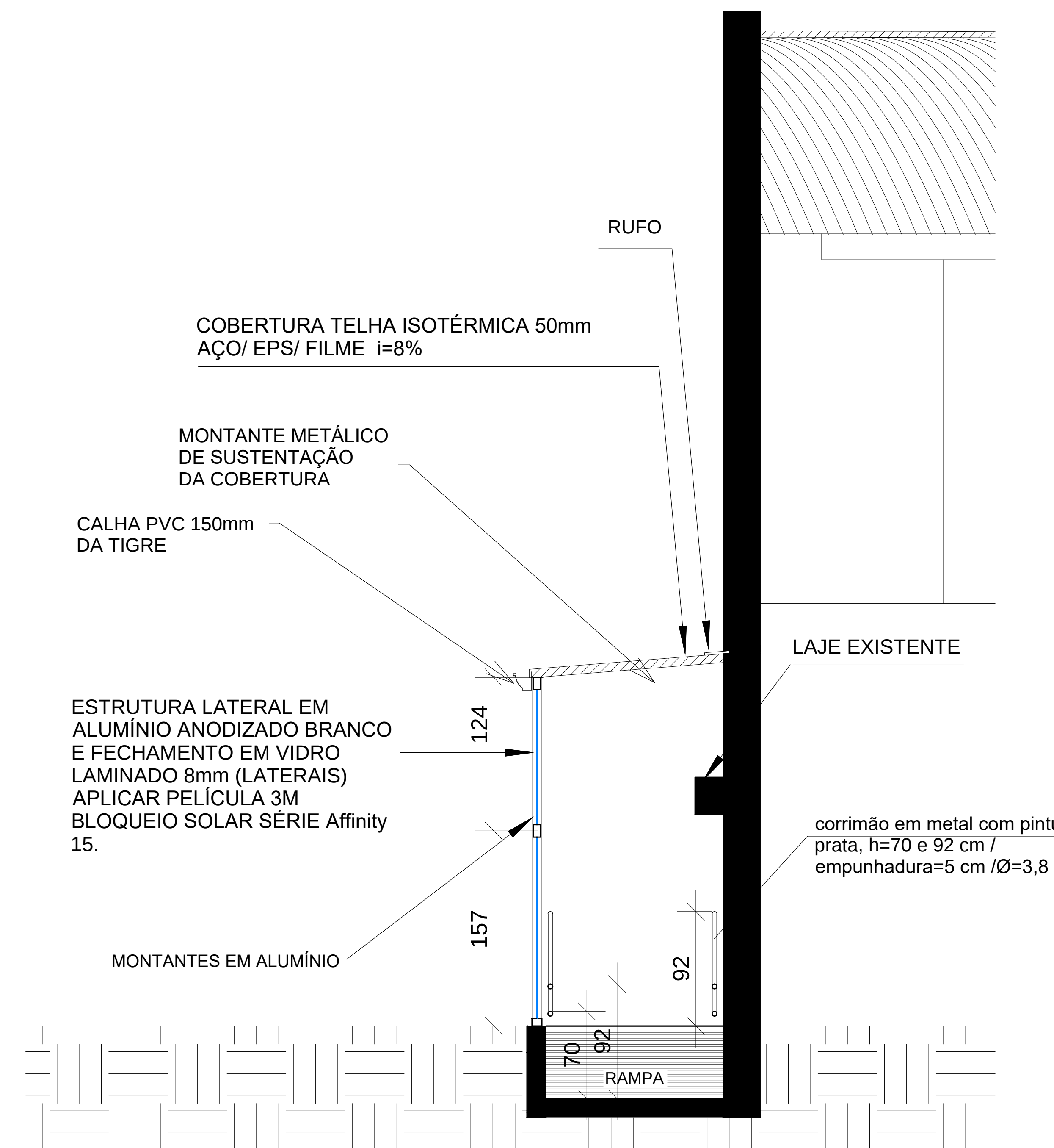
CORTE 2 Escala: 1:25
